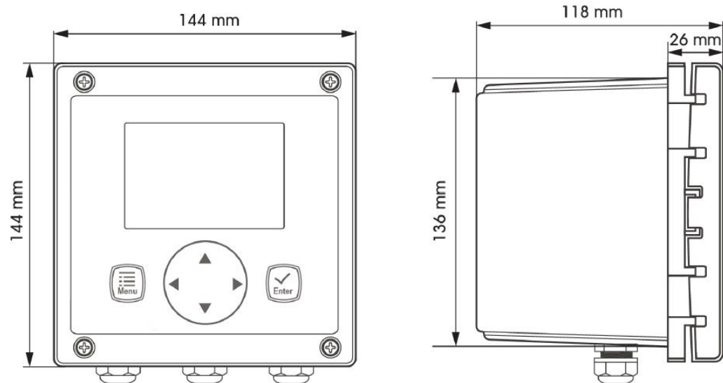
控制器外形尺寸
