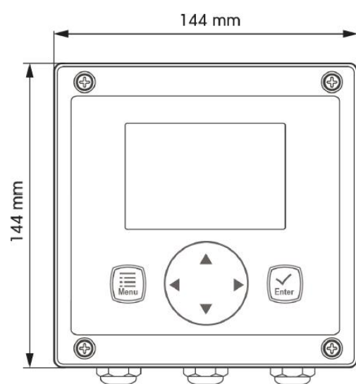
控制器外形尺寸
