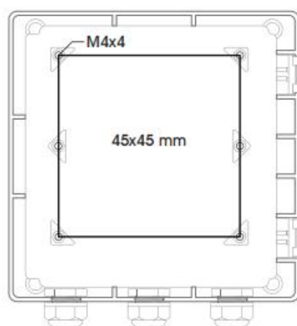
背部固定孔尺寸
